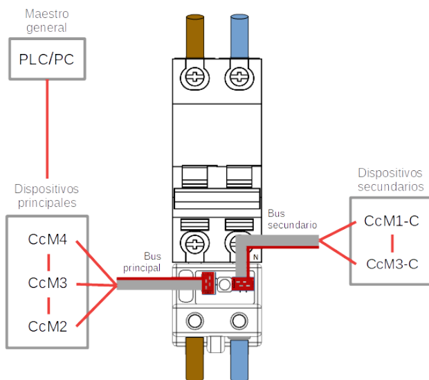
Figura 14 Conexión buses principal y secundario
