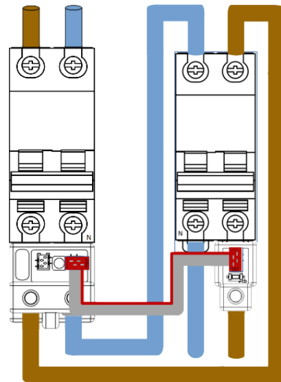
Figura 17 Conexión bus secundario
