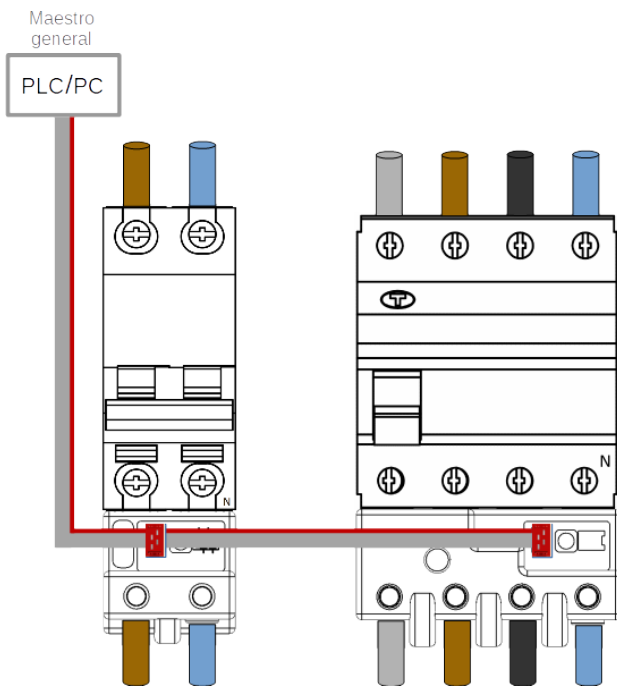
Figura 16 Conexión bus principal CcM2
