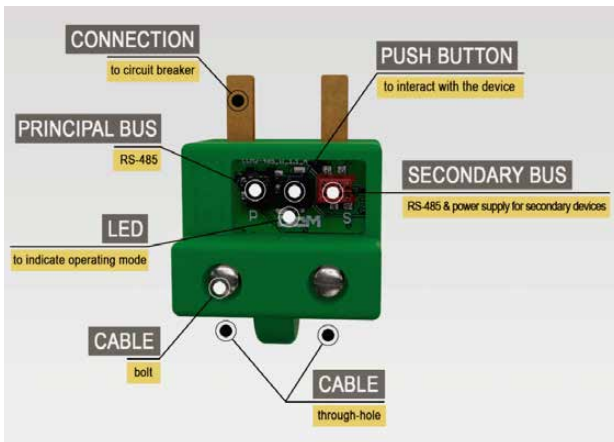
Figura 2 Descripción gráfica CcM2
