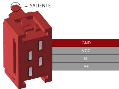
Figura 12 Conector RS-485
