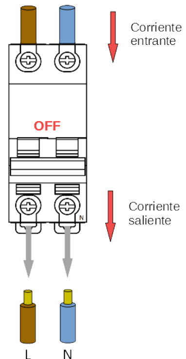
Figura 7 Desconexión de las líneas de corriente
