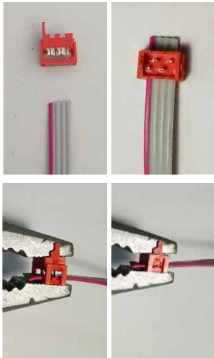
Figura 11 Crimpar conector para cable RS-485
