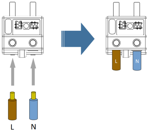
Figura 8 Conexión de cables en CcM2
