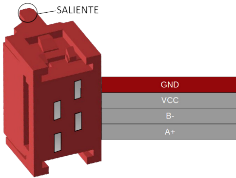
Figura 10 Conector RS-485
