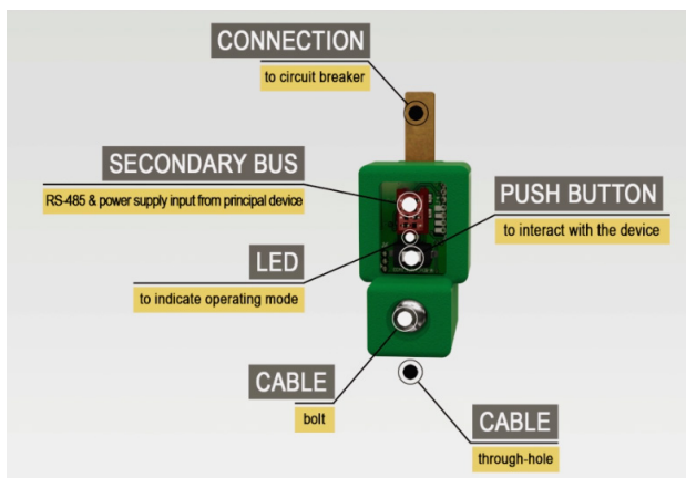
Figura 2 Descripción CcM1-DC
