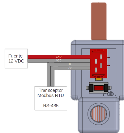
Figura 12 Conexión CcM1-C a transceptor Modbus RTU
