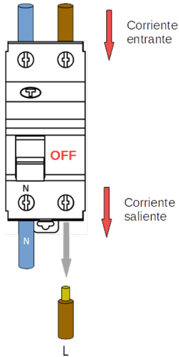
Figura 6 Desconexión de las líneas de corriente
