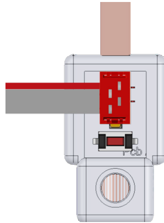
Figura 11 Conexión bus RS-485
