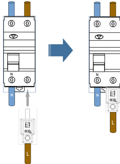
Figura 8 Conexión de CcM2-W a interruptor
