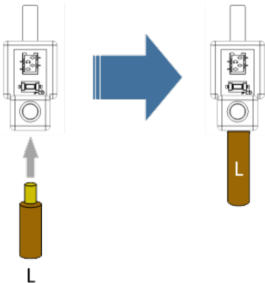
Figura 7 Conexión de cable en CcM1-C
