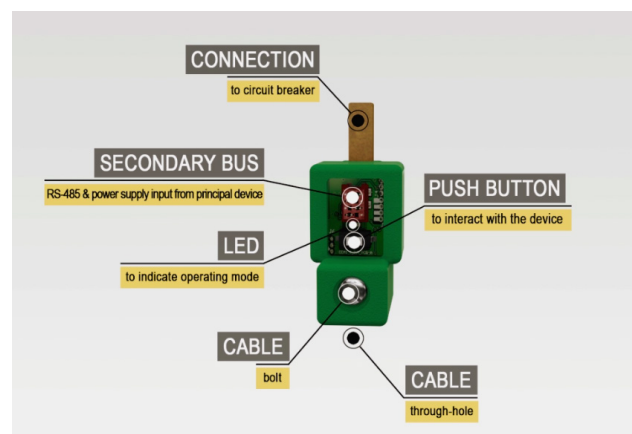
Figura 2 Descripción CcM1-C
