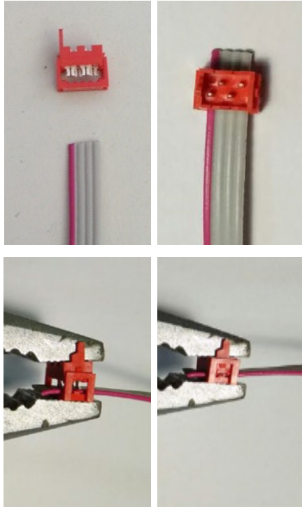
Figura 9 Crimpar conector para cable RS-485
