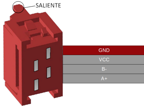
Figura 10 Conector RS-485
