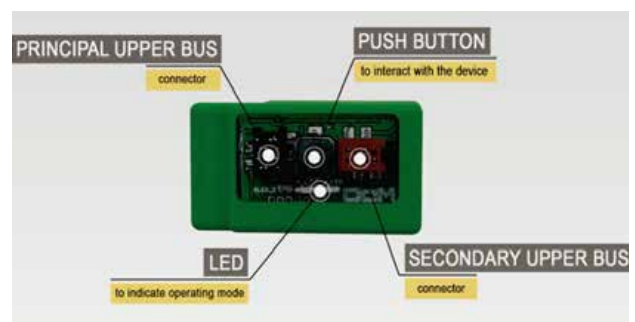
Figura 2 Descripción gráfica CcM WiFi (parte superior)
